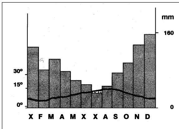
Climograma do golfo Ártabro segundo índice de Gaussen.
