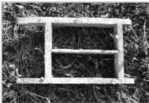
Molde duplo para senlos tixelos macizos.
