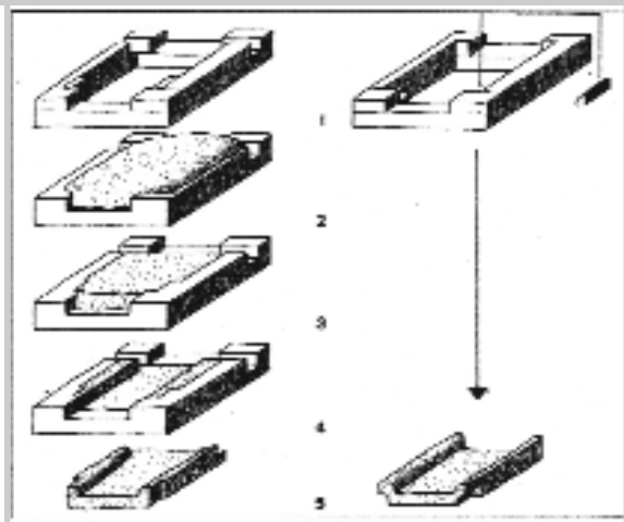
Proposta de molde típico romano para a fabricación de tégalas (Tomado de PÉREZ, 1992: 250, Fig. 3)
