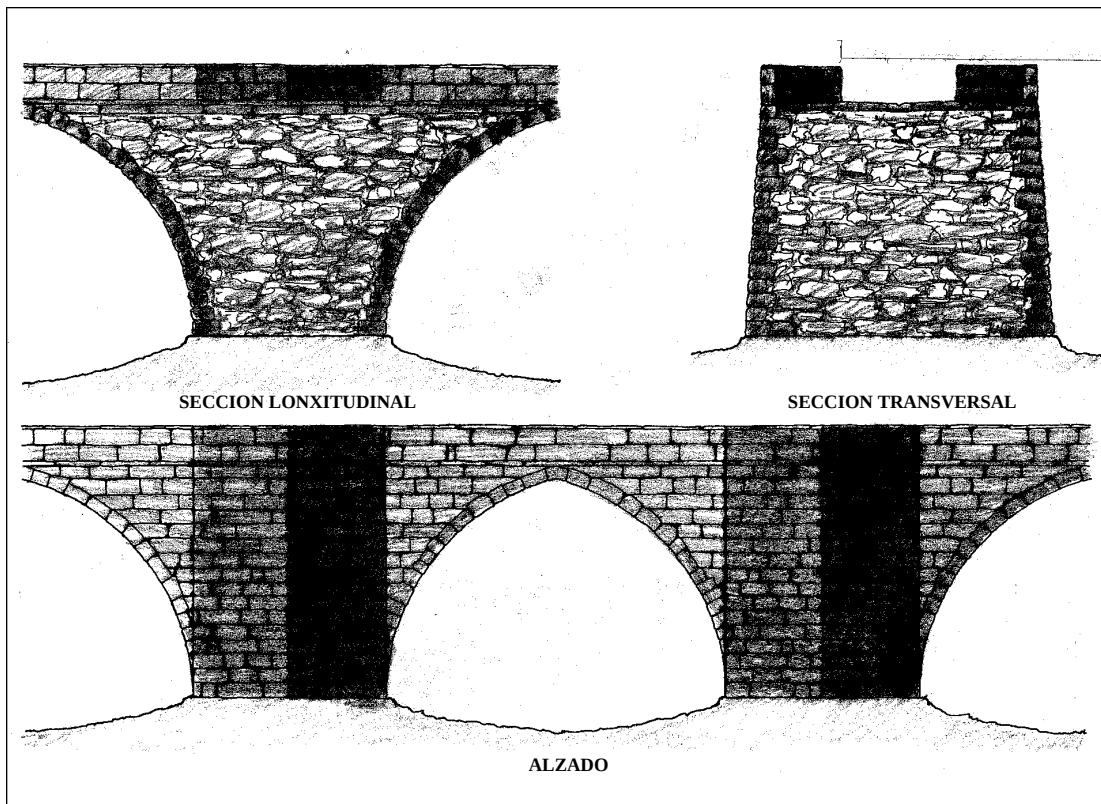
Debuxo 3: Detalle do arco da ponte.
