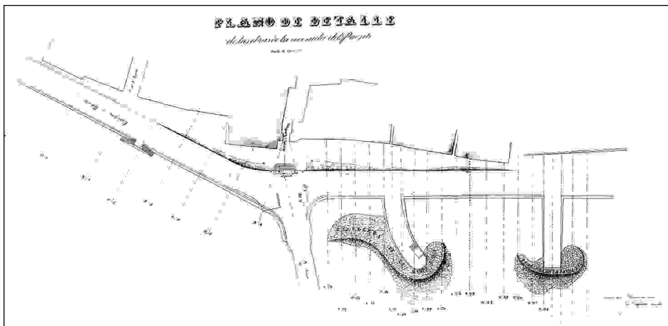
Plano 5. A ponte, a entrada de Pontedeume (AXA).
